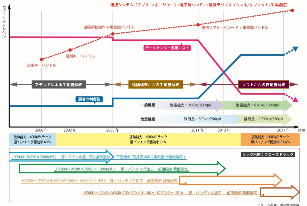
図 30 サーバールックの構造と性能の変遷
