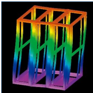
CAEによる振動解析
