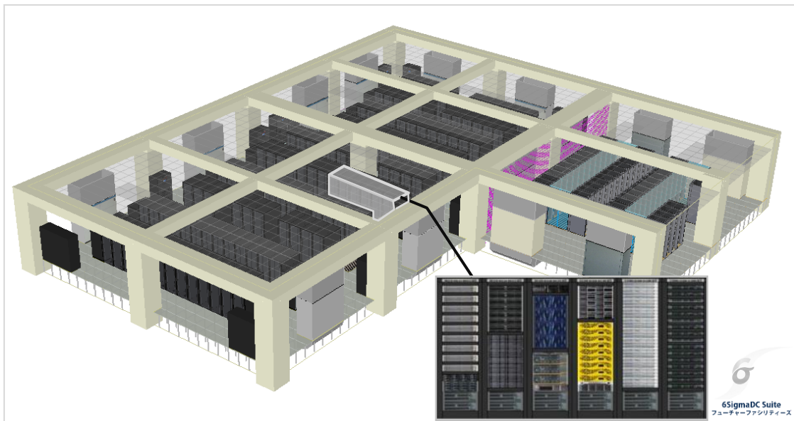
図 16 データセンターの3次元シミュレーションモデル
