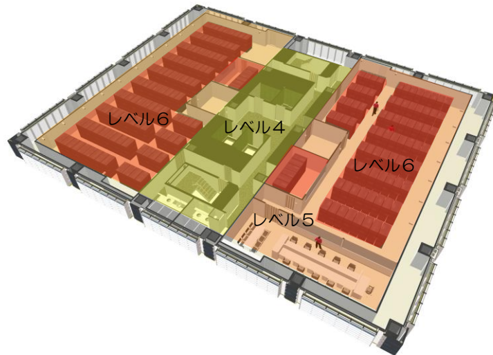
図 15 「架空のデータセンター」サーバー室階のゾーニングイメージ
