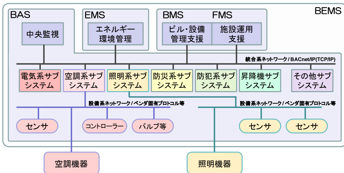
図 6 BEMSの全体イメージ
