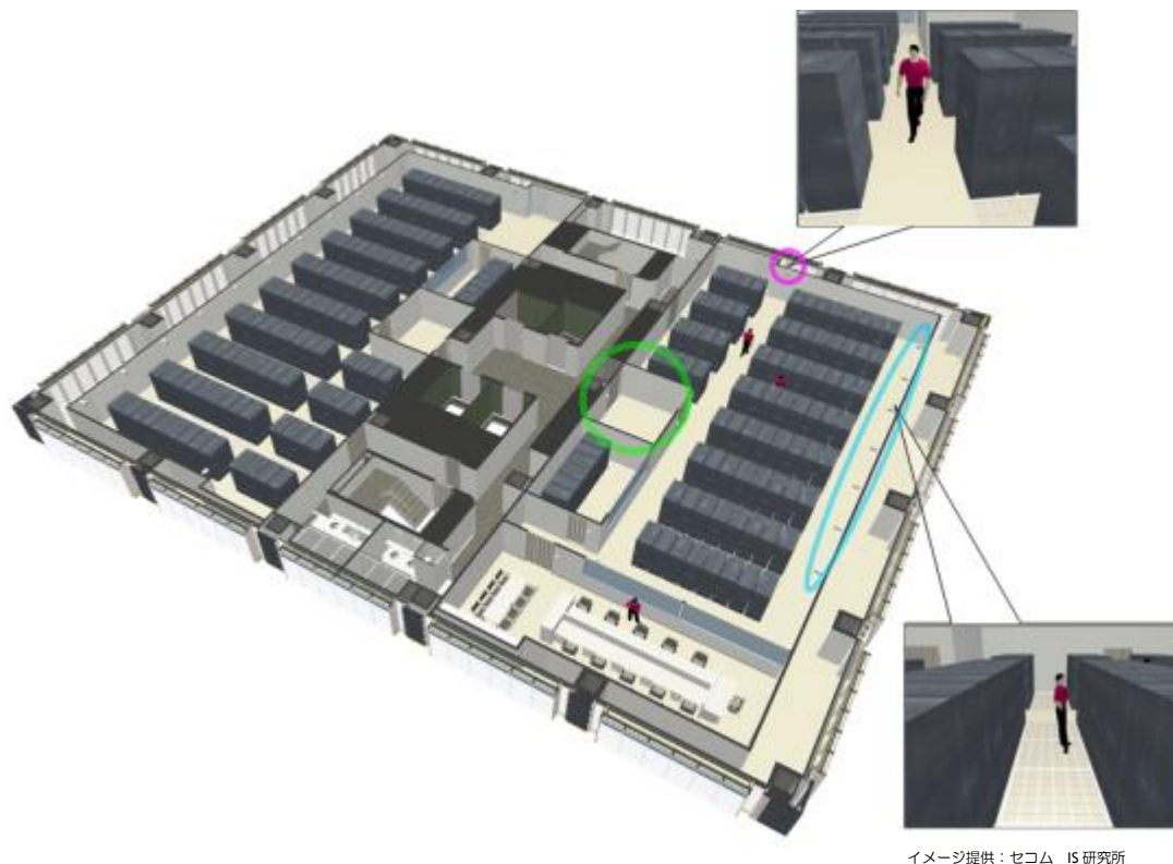
図 19 「架空のデータセンター」におけるサーバー室階部分の管理策
