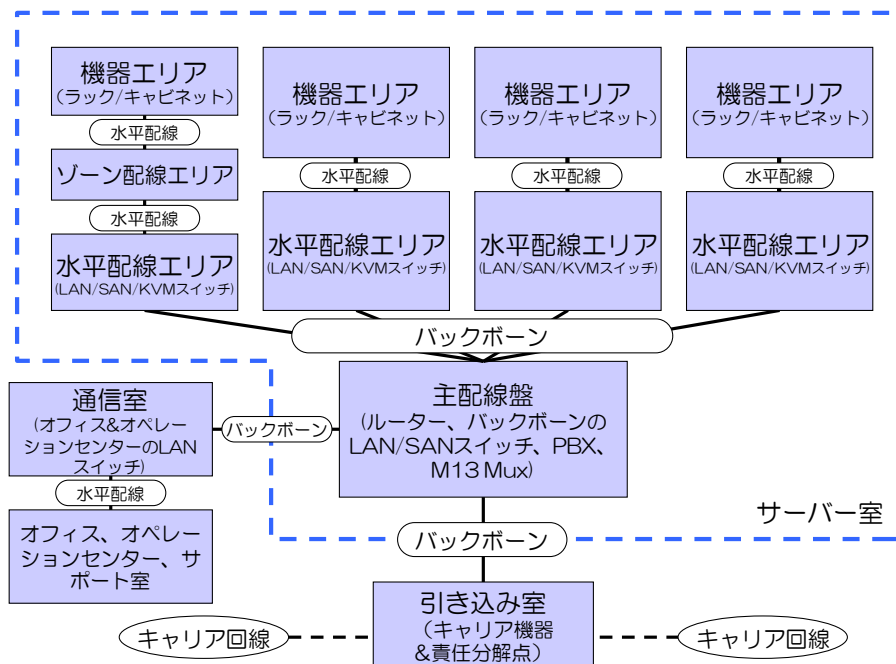
図7 ANSI/TIA-942におけるデータセンターのケーブル配線のモデル
