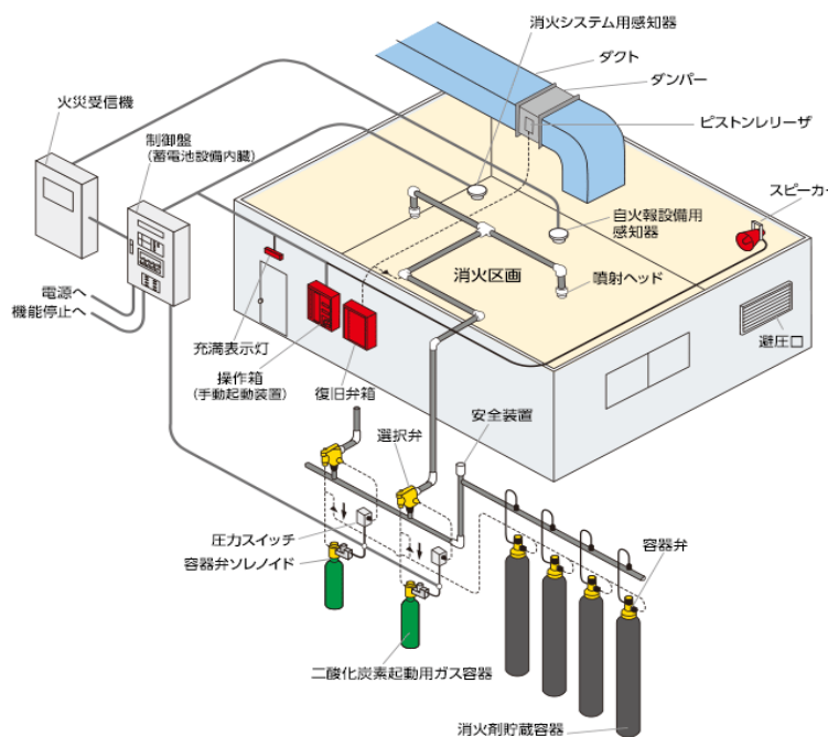
ガス系消火設備のシステム構成例
