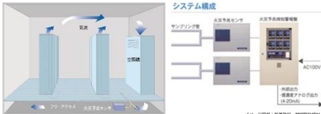
図 27 火災予兆システムの設置方法（左）とシステム構成（右）
