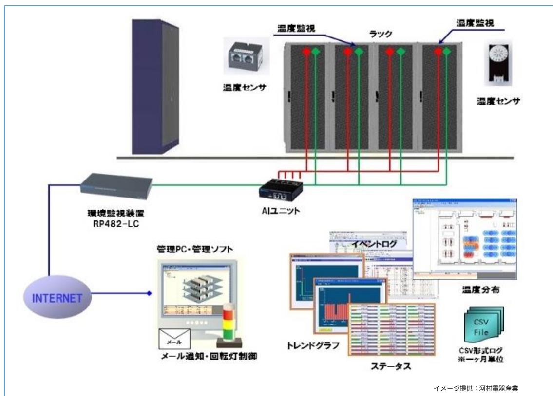
図 25 サーバーラック内温度・湿度監視システムの例
