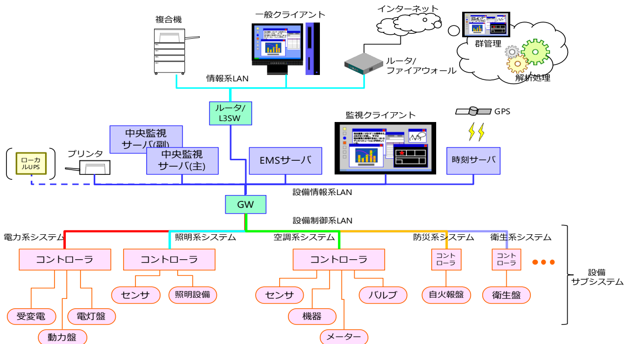
図 36 ビルディングオートメーションシステムの構成
