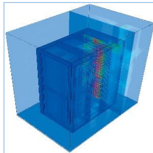
CFDによる熱解析
