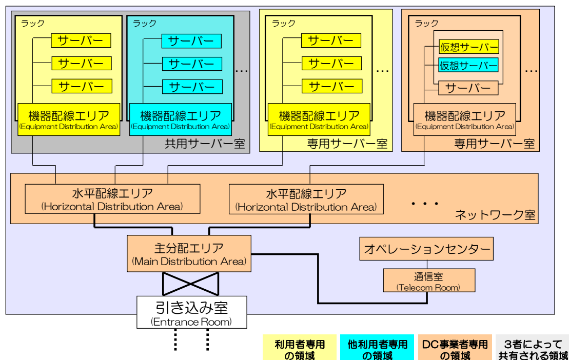
図 8 物理ネットワークと物理セキュリティ区画の関係
