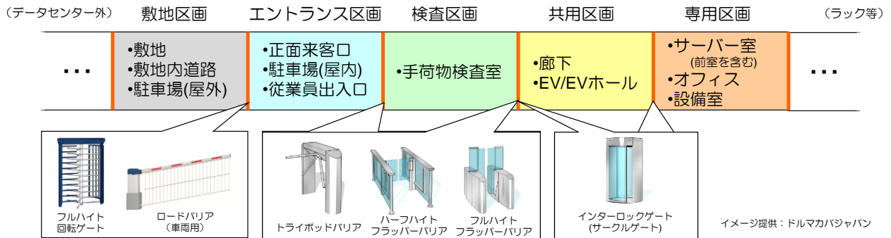
図 29 セキュリティゲートの配置例
