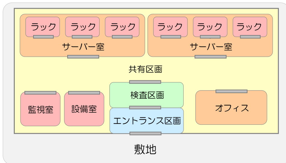
図 5 典型的なデータセンターの空間構造
